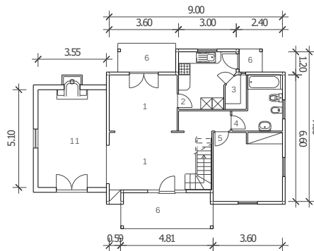
PLANTA DO R/CHÃO R/CHÃO 100.50 m 2
