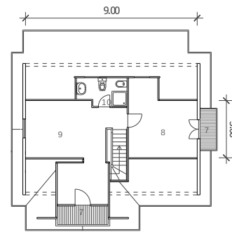
PLANTA DO 1° ANDAR 1° AND. 44.10 m 2
