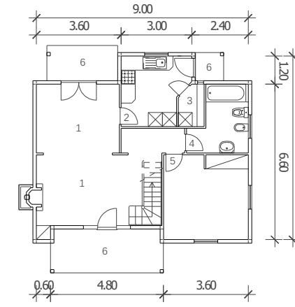
PLANTA DO R/CHÃO R/CHÃO 78.50 m 2
