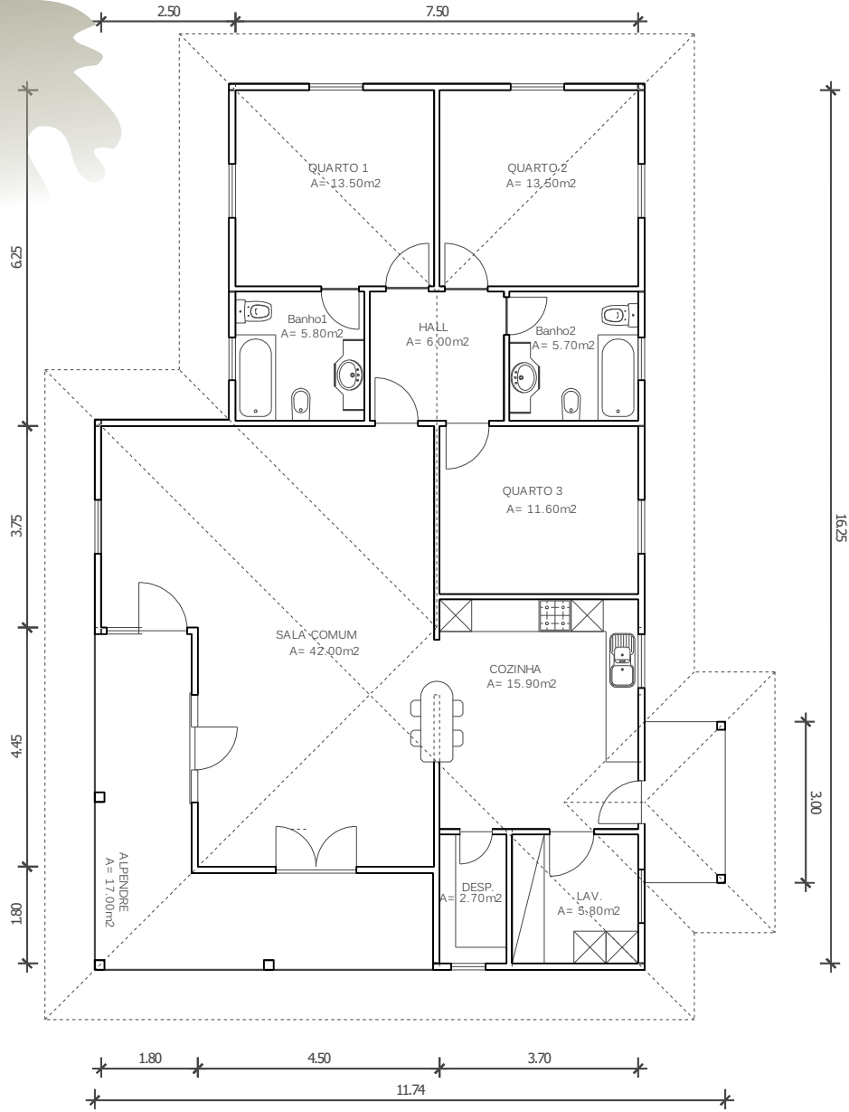
PLANTA
