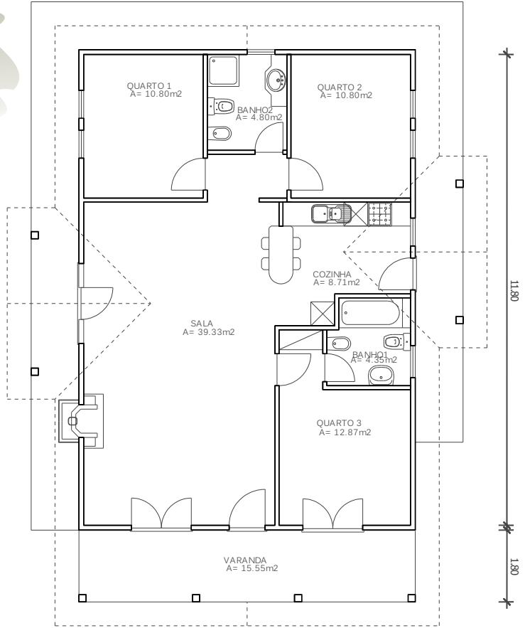
PLANTA
